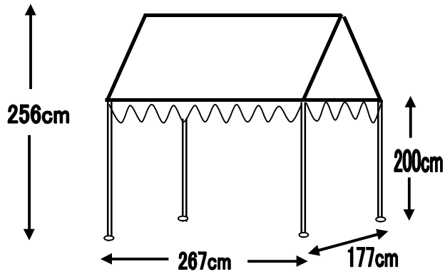
集会用テント 1K×1.5K 約1.5坪(4.72㎡)
