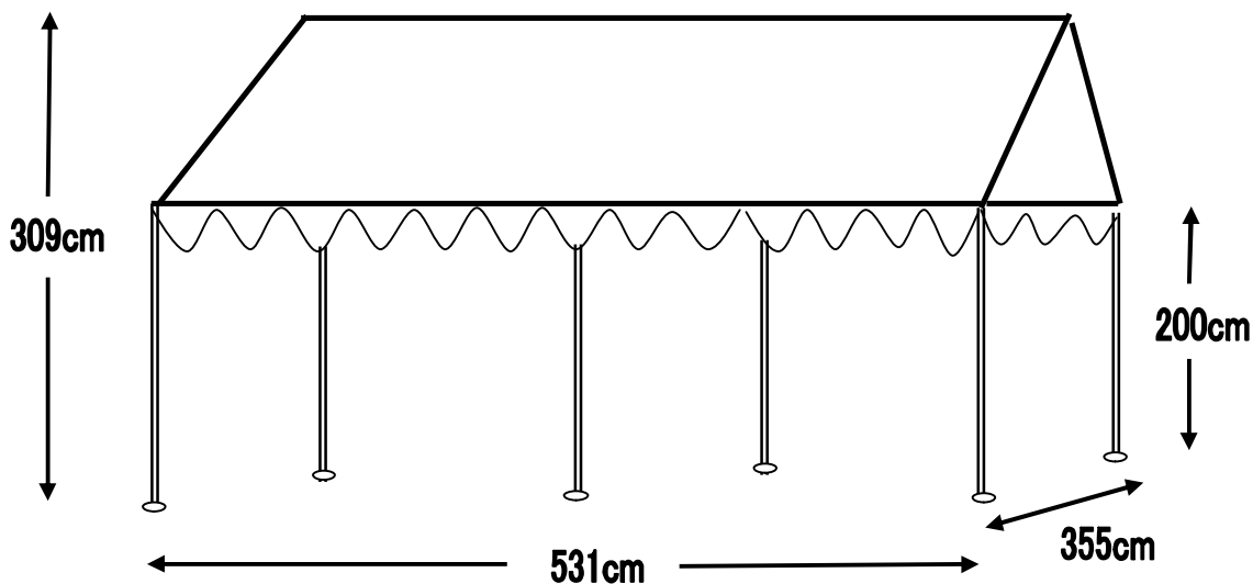
集会用テント 2K×3K 約6坪(18.8㎡)
