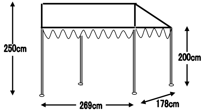
方流れテント 1K×1.5K 約1.5坪(4.80㎡)
