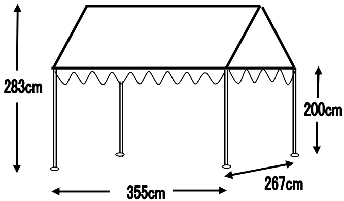
集会用テント 1.5K×2K 約3坪(9.48㎡)
